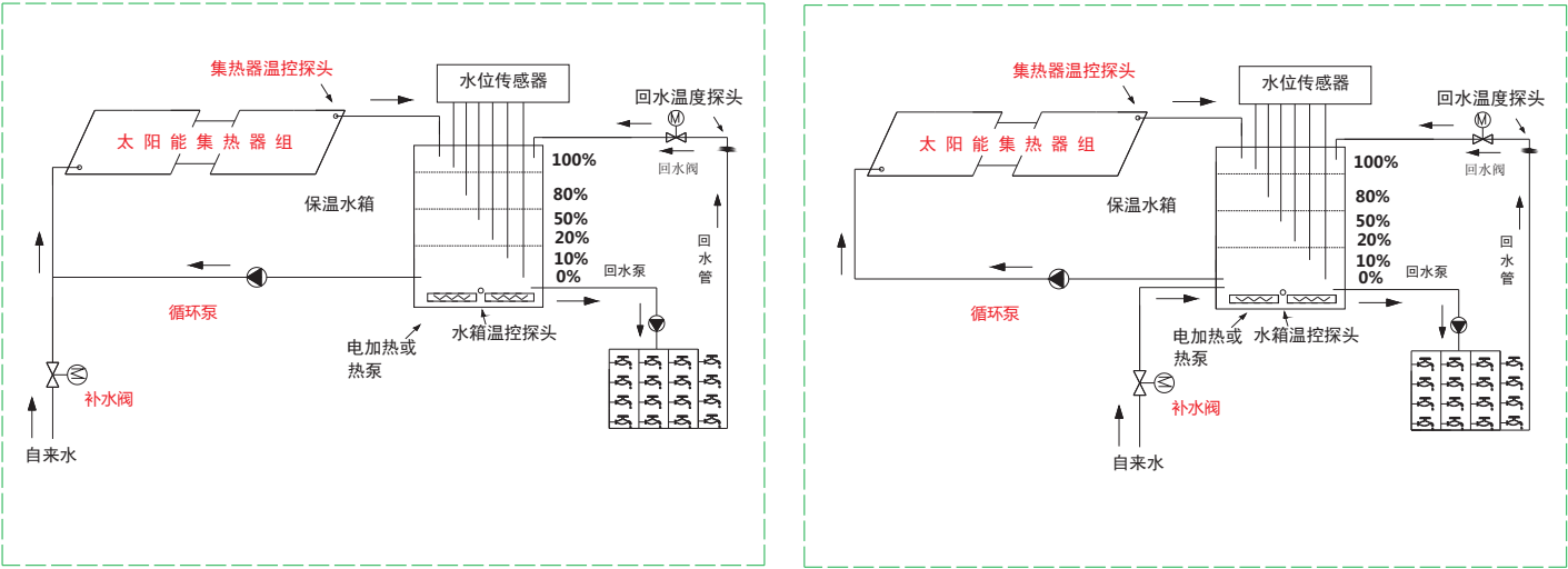
LD-300T工程示意图
